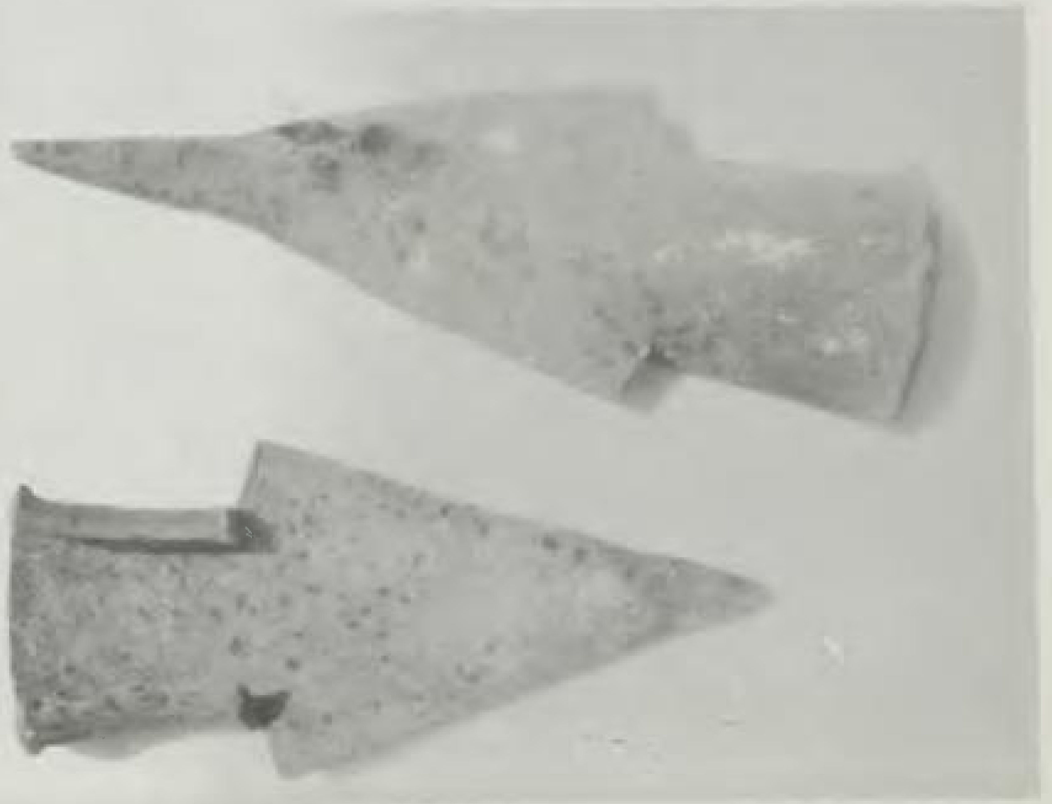
66. Το σιδερένιο υνί για το Ματσουκιώτικο ξυλάλετρο (28-8-1993).
